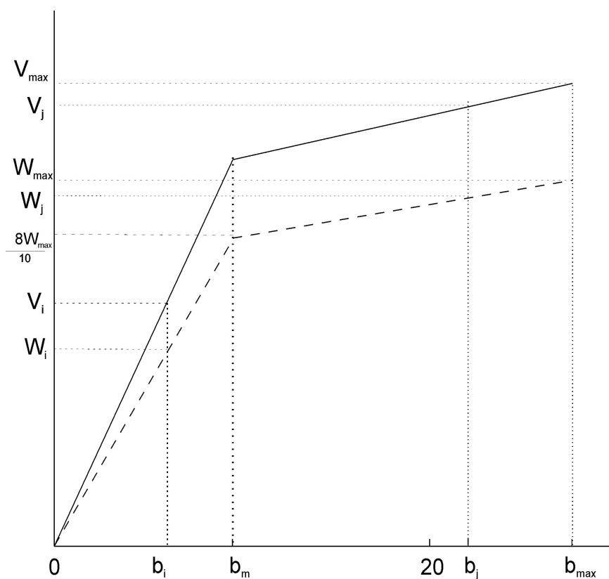
Figura 2: Representación gráfica das puntuacións se b_{max} > 20 .
